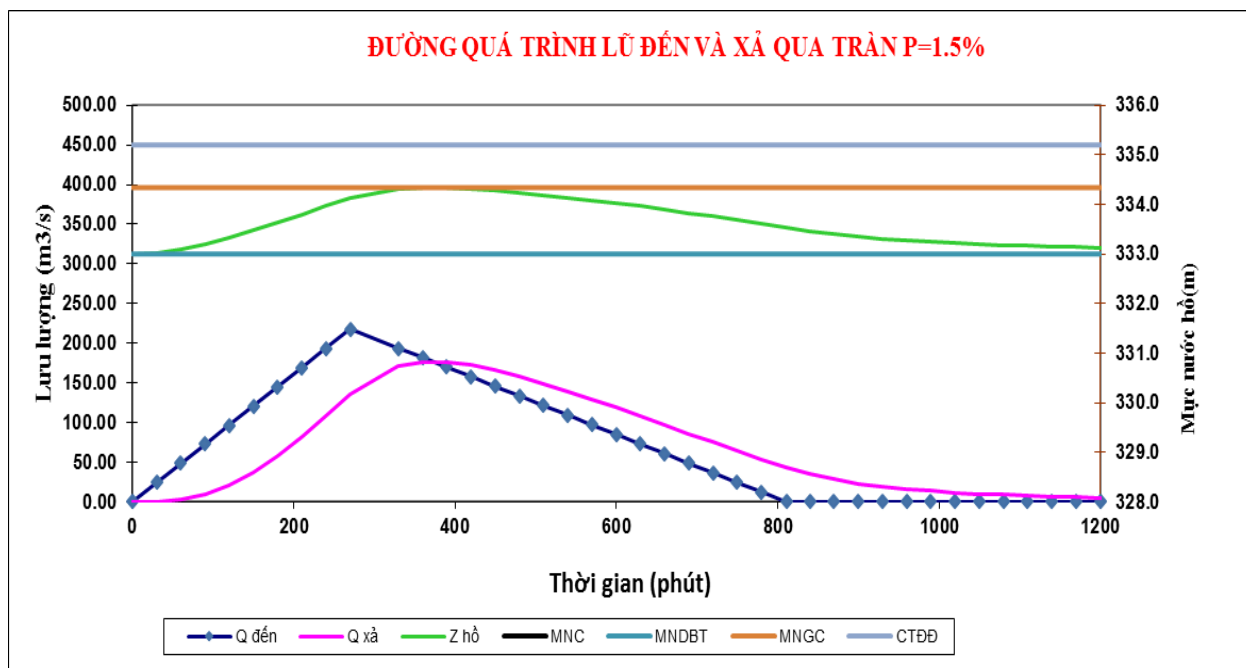
Biểu đồ điều tiết lũ thiết kế (P=1,5%)
